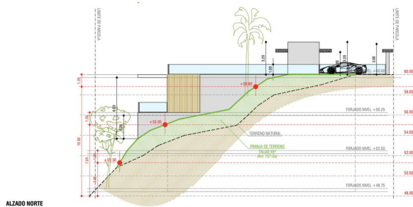
ALZADO NORTE
